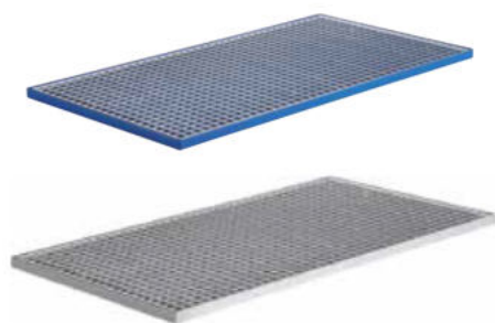
Typ: 7560 / 7560-Z Záchytná podlaha na skladovanie sudov a nádob s kvapalinami
